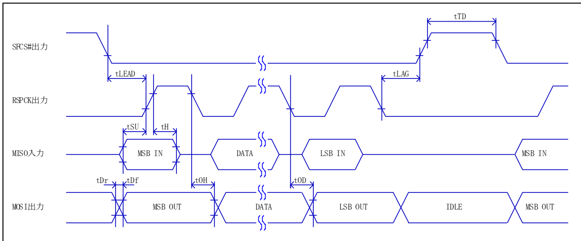
图 4-4 SPI 时序 (SPI 模式 模式 0)
