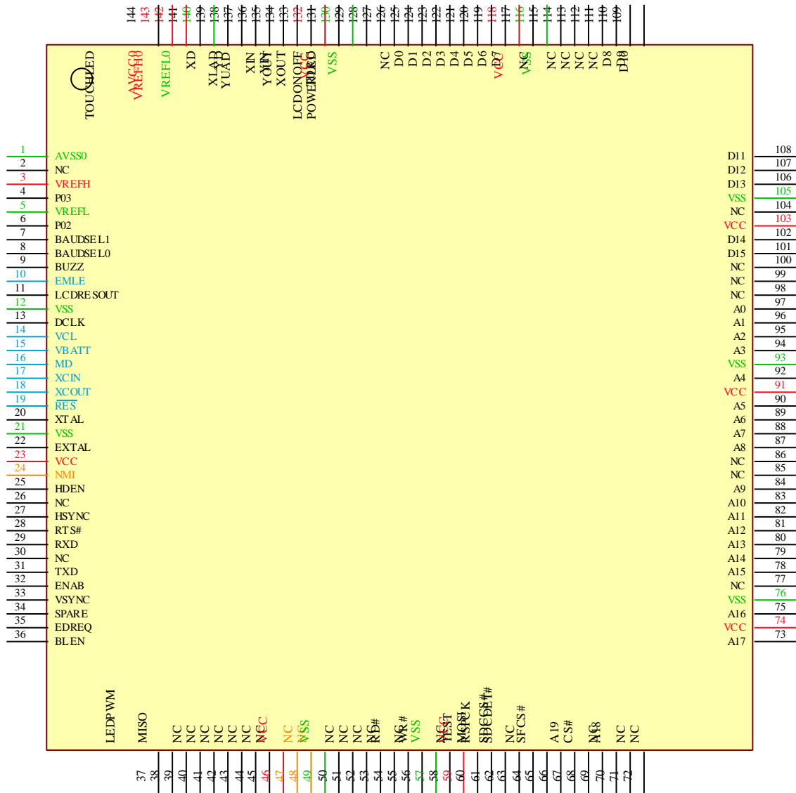
图 3-1 KS-430CT-I1 引脚布局图
