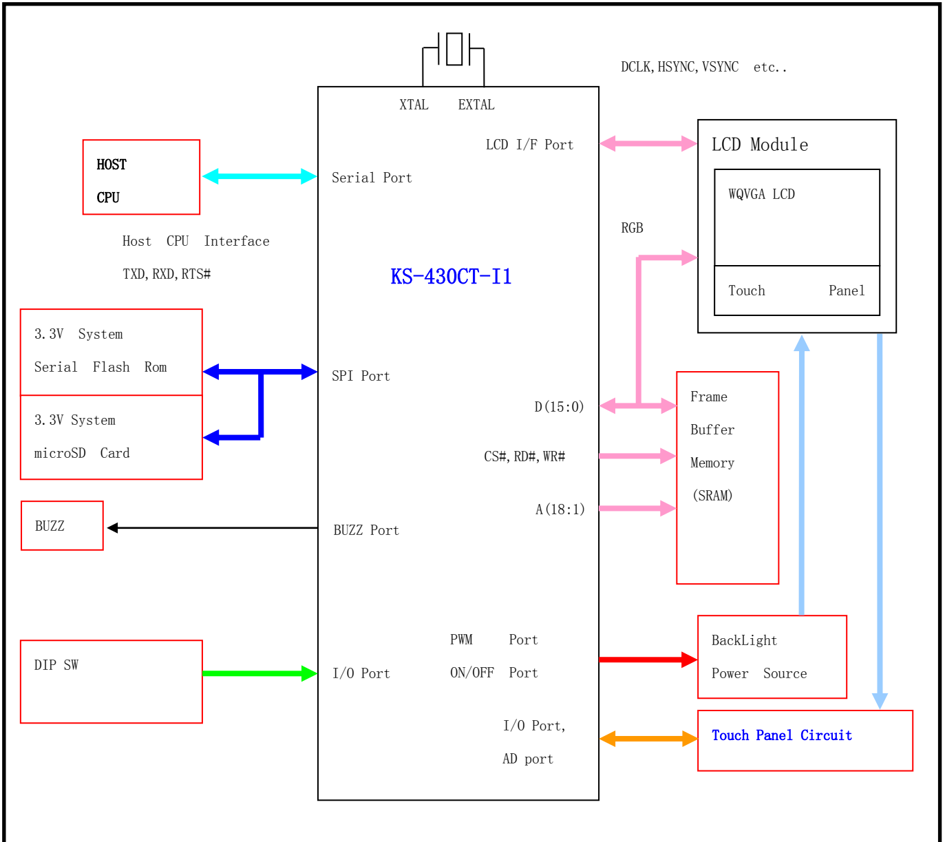
图 2-1 方框图
