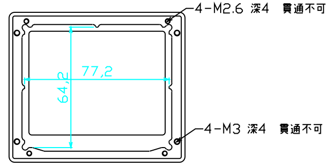
フレーム A5052 t6.0
